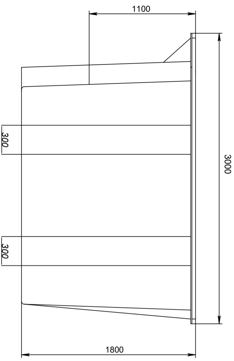
Вид 1-1
