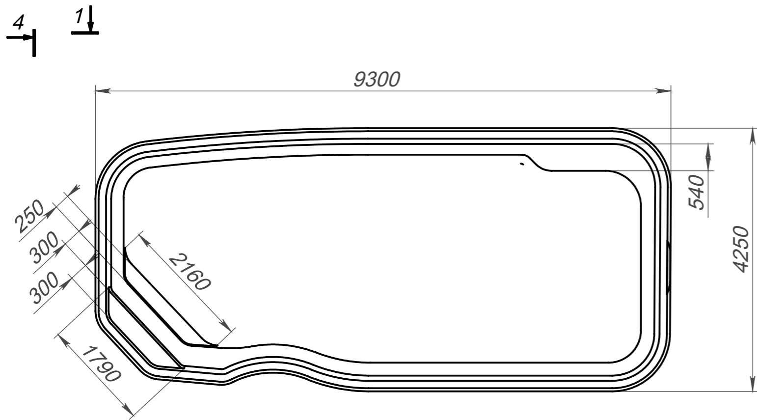
Вид 1-1
