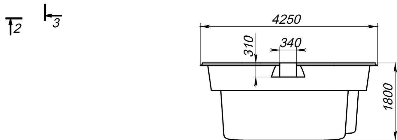
Вид 3-3
