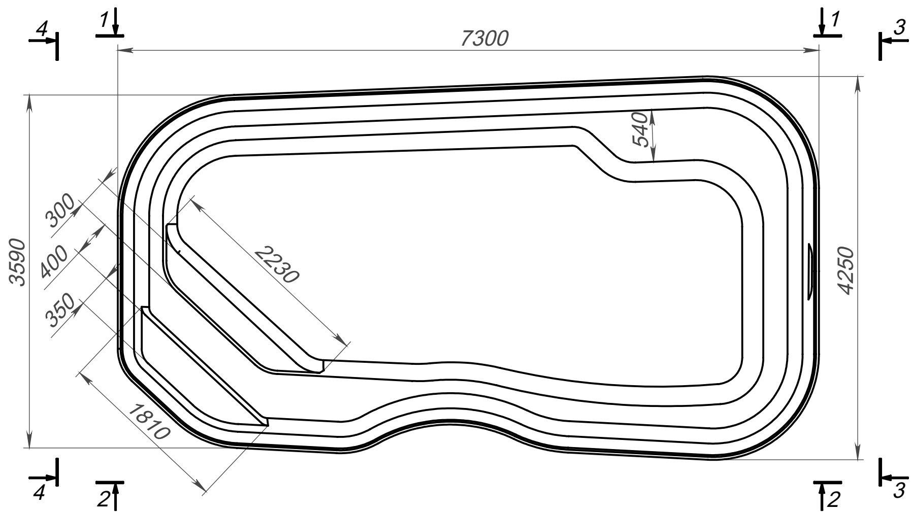
Вид 1-1
