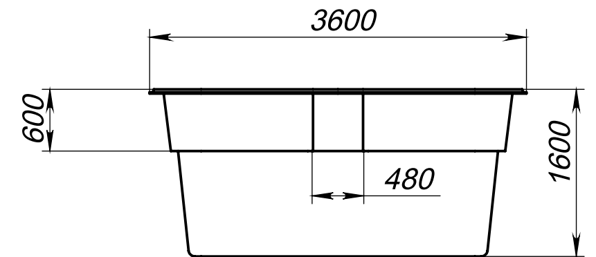
Вид 3-3
