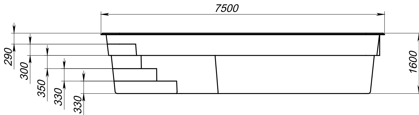
Вид 2-2
