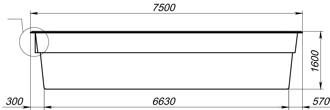
Вид 1-1
